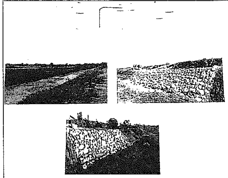
Imagen 3. Recubrimiento con piedra en tramos de cambio de dirección del flujo"
